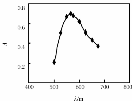
图 1 Se 的光谱扫描曲线
