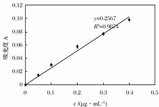
图 2 Se 的标准曲线
