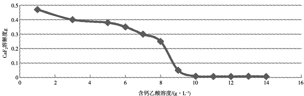
图 1 CaF 2 溶解度与含钙乙酸浓度关系图
